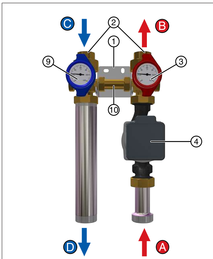
Fig. 5: Vista de conjunto de los componentes HK25 y HK32
