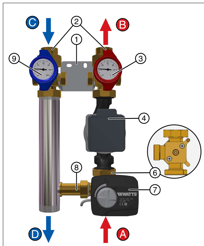
Fig. 6: Vista de conjunto de los componentes HKM25 y HKM32
