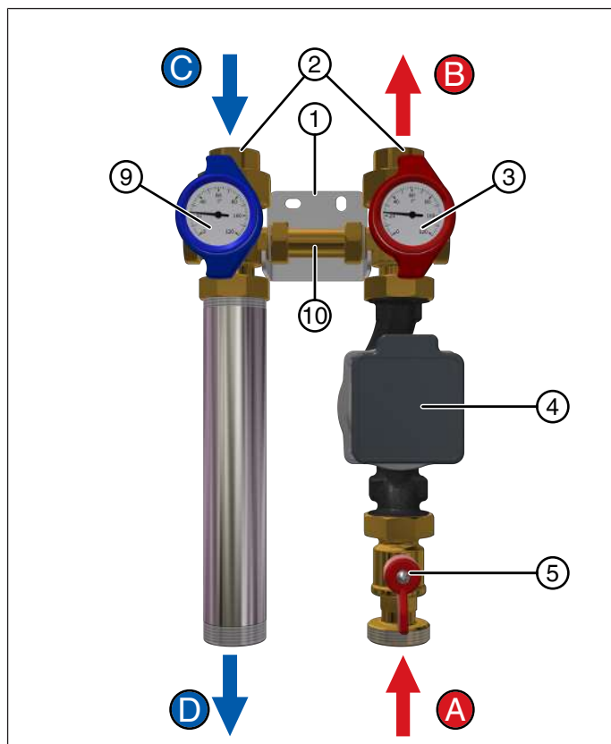
Fig. 7: Vista de conjunto de los componentes HK25-KH
