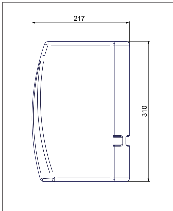
Rys. 4: Łupina izolacyjna grup pompowych FlowBox DN20
