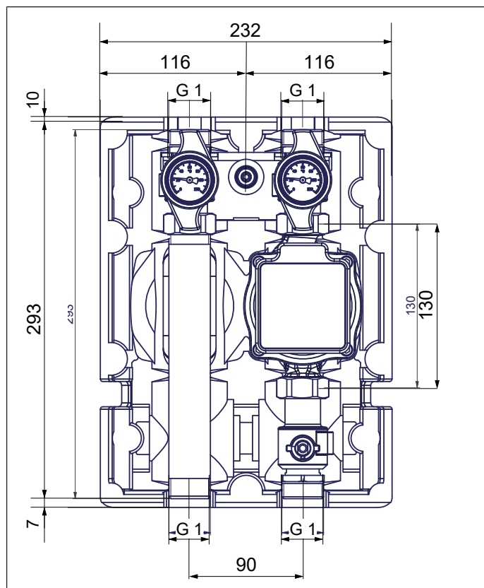
Rys. 3: Grupa pompowa z dodatkowym zaworem kulowym HK20-KH
