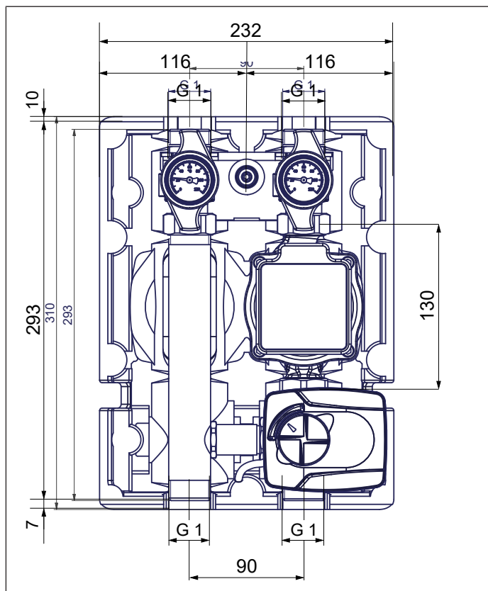
Rys. 2: Grupa pompowa z mieszaczem HKM20
