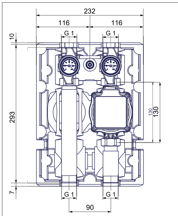
Rys. 1: Grupa pompowa HK20
