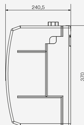
ИЗОЛЯЦИОННЫЙ КОЖУХ FLOWBOX DN 25/32
